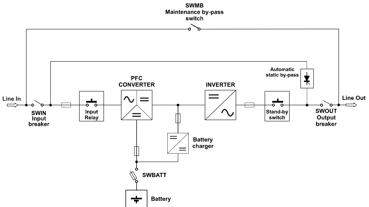
Blockscha der USV
