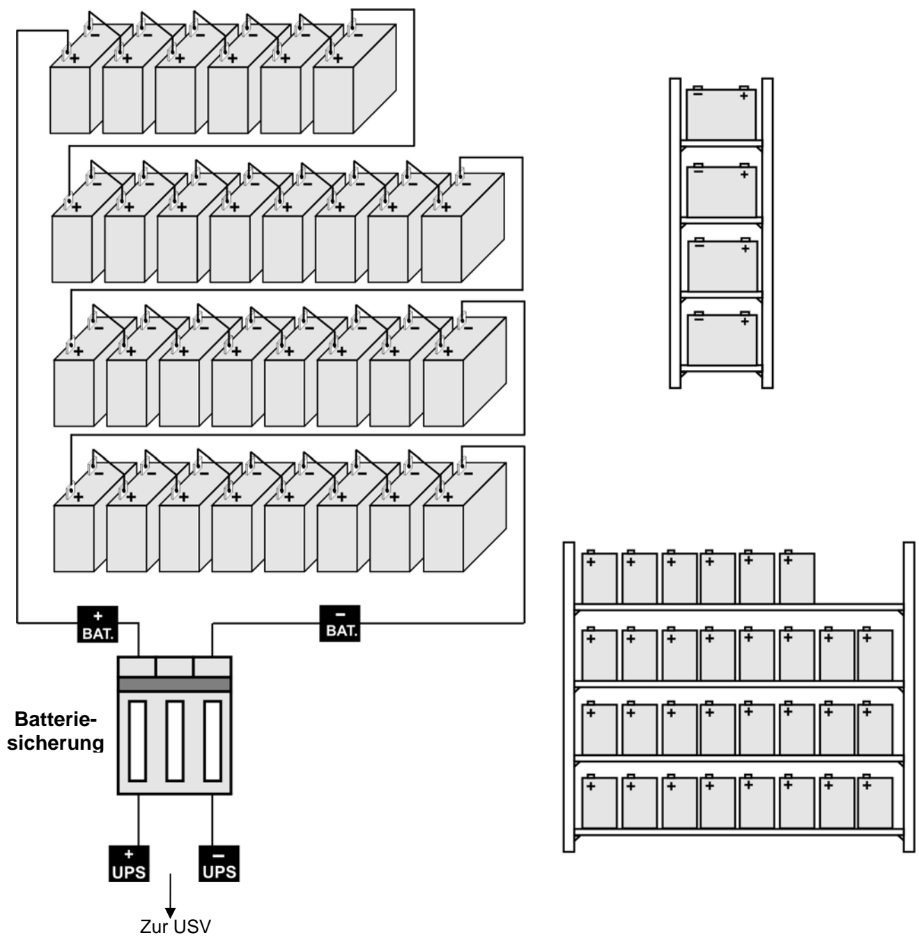
Bild 5-5-a USV-Batterie-Anschluss mit Batteriesicherung
