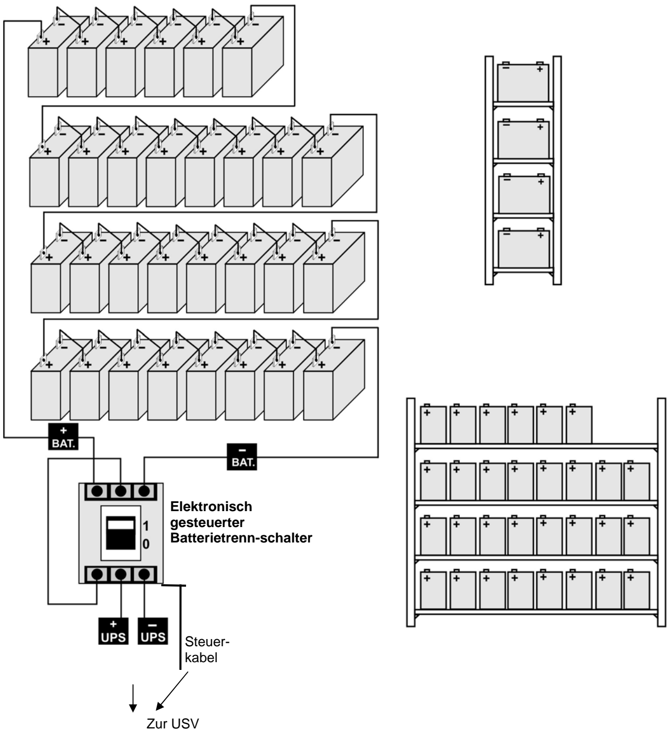
Bild 5-5-b USV-Batterie-Anschluss mit Batterietrennschalter
