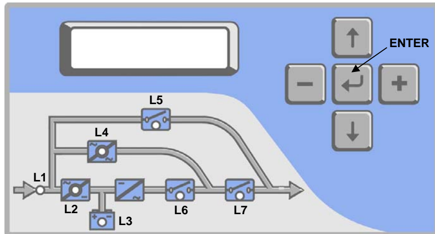
Bild 2-1-a Bedien- und Anzeigefeld (100-120 kVA)
