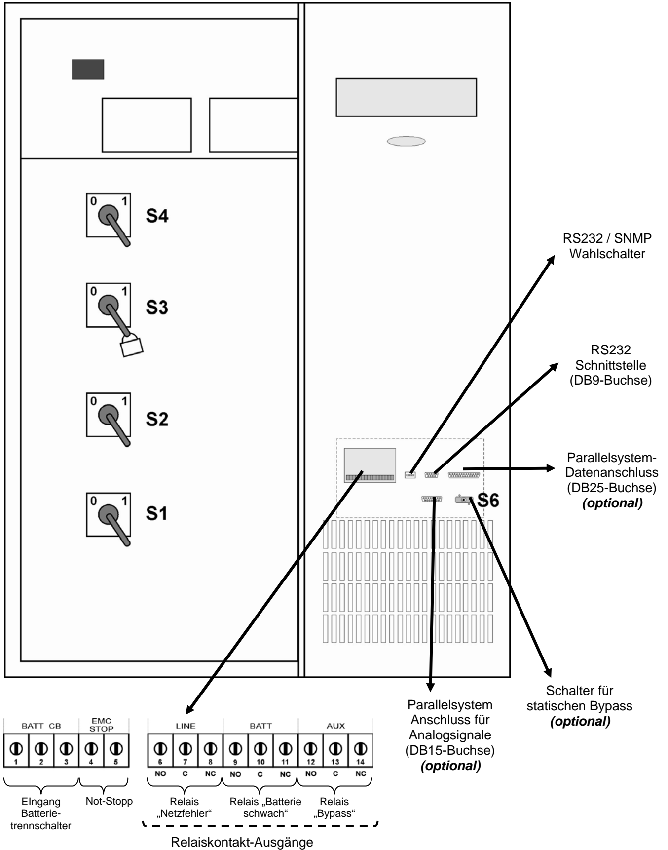
Bild 1.3 100-120-150-160-200 kVA Leistungsschalter
