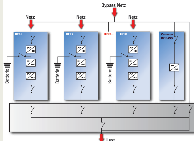
Parallelkonfiguration von bis zu 8 Einheiten mit zentralem Bypass
