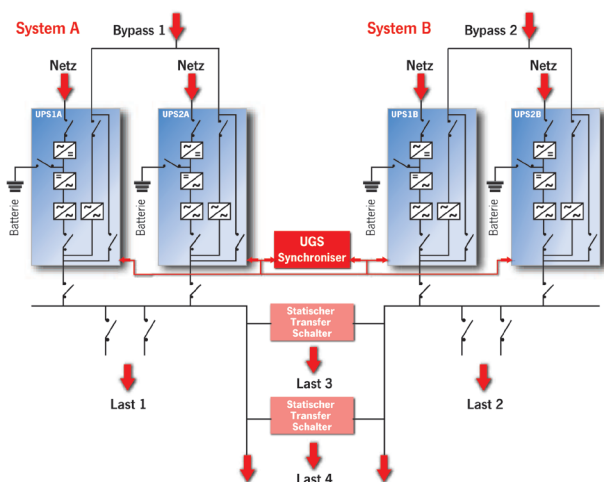
Dynamische Konfiguration Dual Bus
