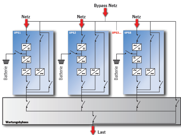
Parallelkonfiguration von bis zu 8 Einheiten mit verteiltem Bypass
